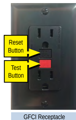
GFCI Receptacle
