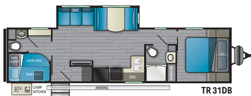
TR 31DB
