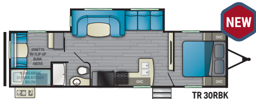
TR 30RBK
